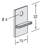
VA 8090 Aufhängeclip mit Öse, Kunststoff
