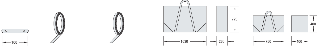
VA 5000 Verbinder gerade (VPE 2 Stück)
